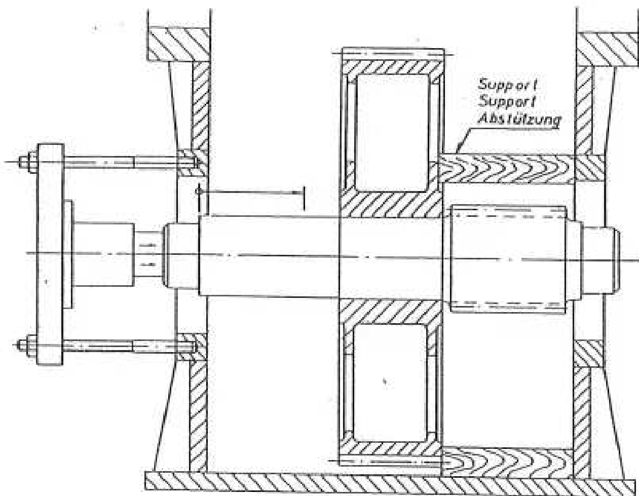
Dismantling - Demontage - Ausbau
