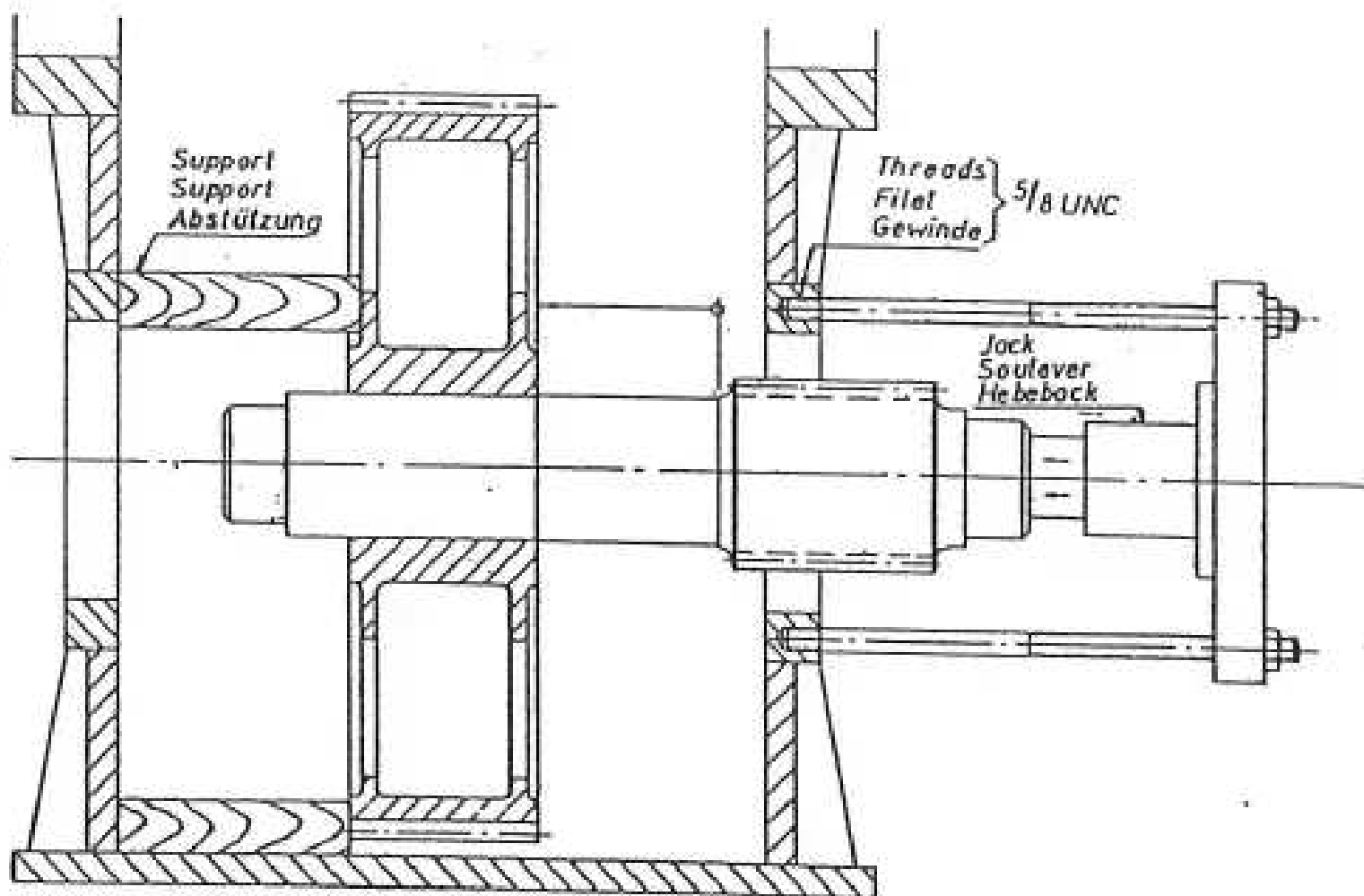
Replacing - Montage - Einbau
